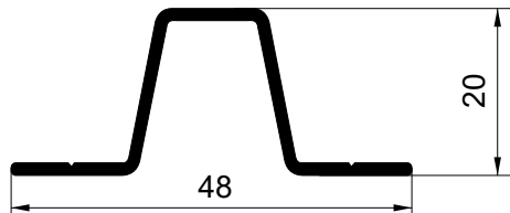
N-1285 0,280 kg/m
