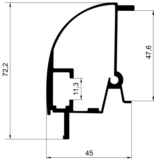
GS-NVC-HB02-002 1,064 kg/m
