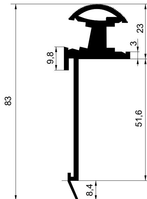
GS-PERFIL 3 1,096 kg/m
