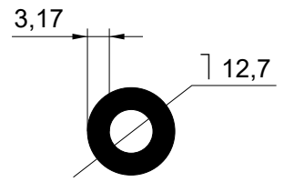
TUB-012 0,258 kg/m
