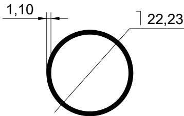
TUB-036 0,181 kg/m
