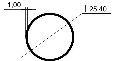
TUB-044 0,208 kg/m
