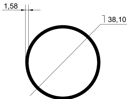
TUB-069 0,494 kg/m
