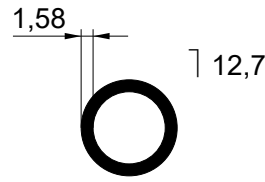
TUB-010 0,150 kg/m
